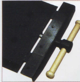
追加鉄製バイス (別の部分や別の作業台に 取り付けられます。) 品番 33461
