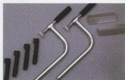
アクセサリキット (ST03、バイスピン(4)、 アルミ製バイスカバー(2)) 品番 33619
