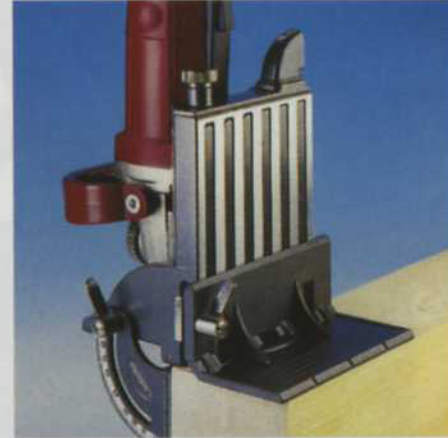
ストップスコヤは、ベースプレートにも取り付け、安定した状態で溝加工ができます。
