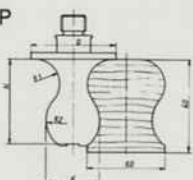
HSSルータービットFRP
